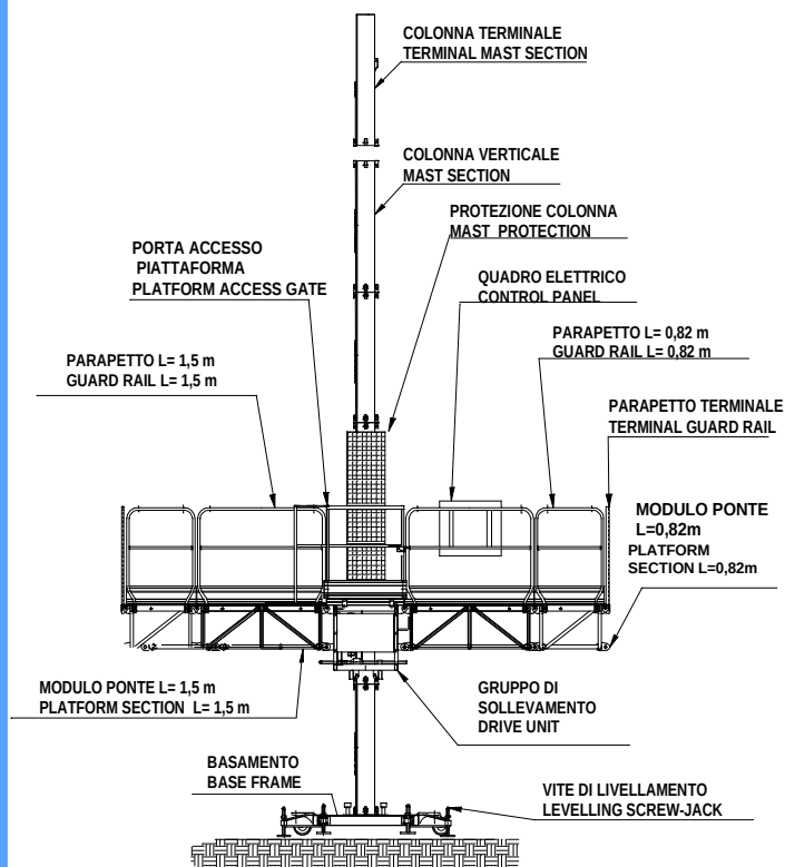
Intervallo ancoraggi Mast tie interval Min/Max 3/7.5 m Altezza libera oltre ultimo ancoraggio Max 6 m Overhang condition
